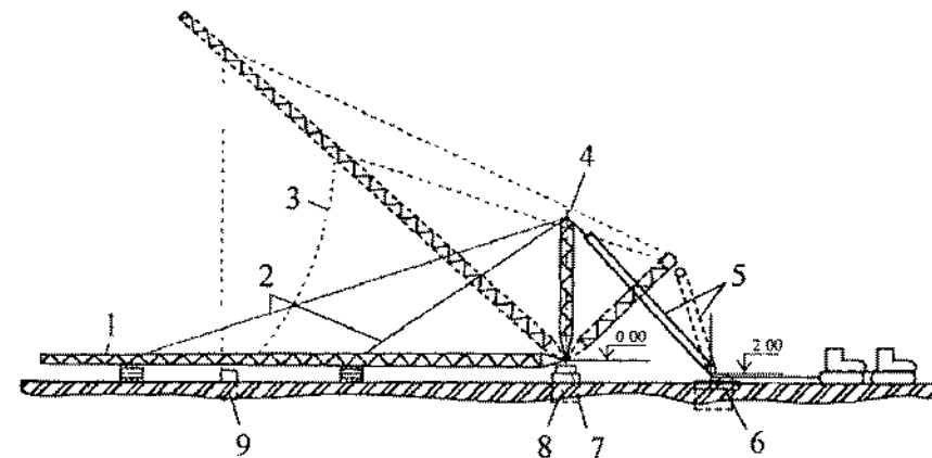
Рис. 16.11. Монтаж мачты методом поворота вокруг шарнира:
