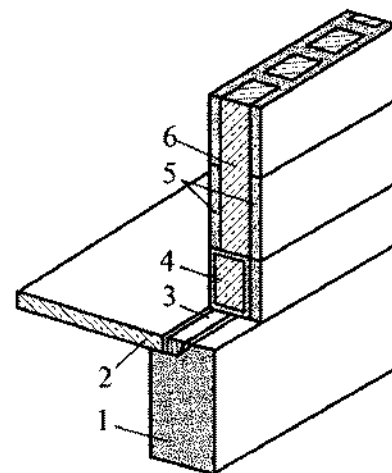
Р и с. 25.5. Сопряжение перекрытия с надстраиваемой стеной:
