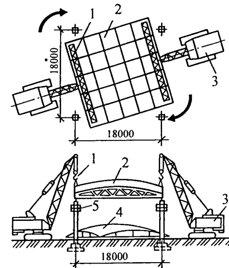
Рис. 8.6. Установка оболочки на опоры методом вертикального подъема:
