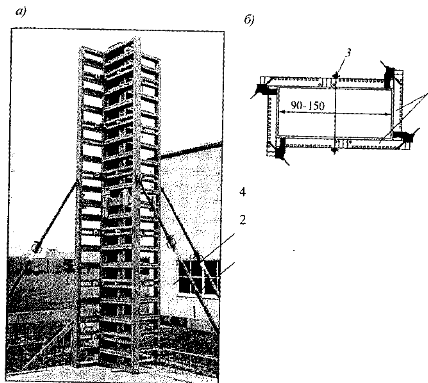
Р и с. 22.8. Опалубка колонн фирмы «НОЕ»:
