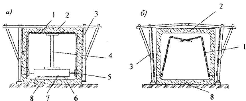
Рис. 23.1. Катучая опалубка для бетонирования подземных коллекторов: а — установка опалубки; б — распалубливание; 1 — внутренняя опалубка; 2 — бетонированный коллектор; 3 — наружная опалубка; 4 — центральная стойка; 5 — домкрат; 6 — катки; 7 — тележка; 8 — днище коллектора
