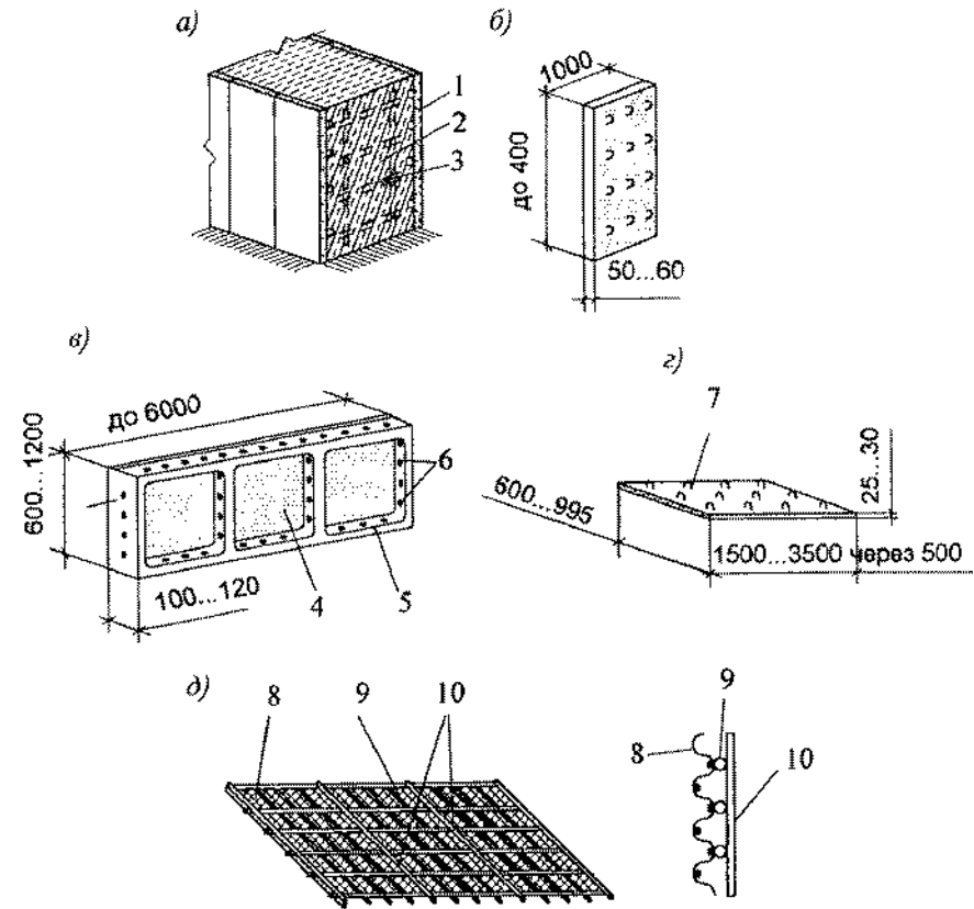
Рис. 25.1. Несъемная опалубка:
