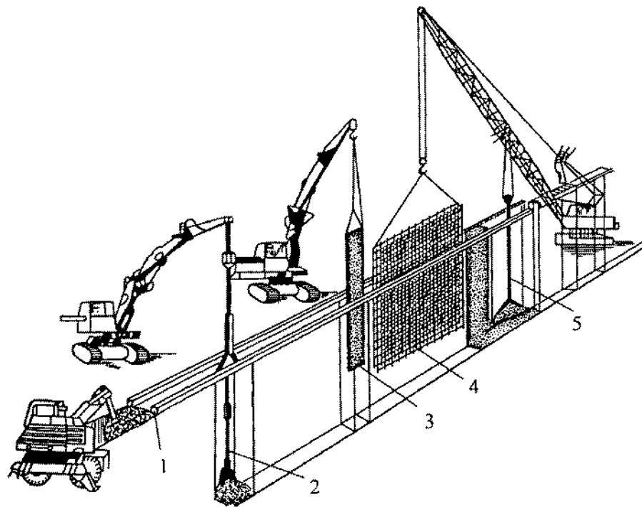
Рис. 6.1. Технологическая схема устройства «стены в грунте»: 1 — устройство форшахты (укрепление верха траншеи); 2 — рытье траншеи на длину захватки; 3 — установка ограничителей (перемычек между захватками); 4 — монтаж арматурных каркасов; 5 — бетонирование на захватке методом вертикально перемещаемой трубы
