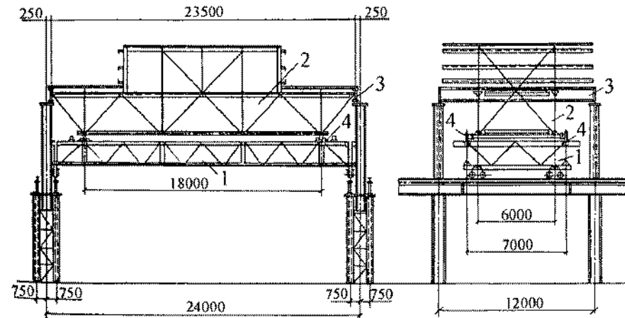
Р и с. 10.8. Установщик для подачи и монтажа блоков:
