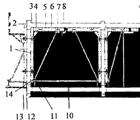
Рис. 23.5. Туннельная опалубка фирмы «НОЕ»:
