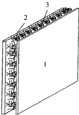
Р и с. 26.5. Виброизоляционный рулонный материал: 1 — геотекстиль; 2 — гидроизо- ляционный слой; 3 — пласт- массовые пружинки
