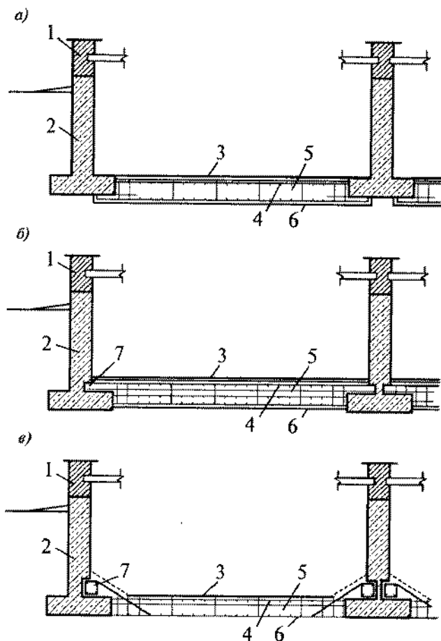
Р и с. 29.6. Варианты переустройства ленточных фундаментов в плитные: а — сплошная плита снизу фундаментных подушек; б — сплошная плита с балками на шпонках; в — сплошная плита на шпонках; 1 — кирпичная стена; 2 — фундамент; 3 — отметка верха пола подвала; 4 — рабочая арматура плиты; 5 — монолитная плита; 6 — подготовка под монолитную плиту; 7 — штрабы
