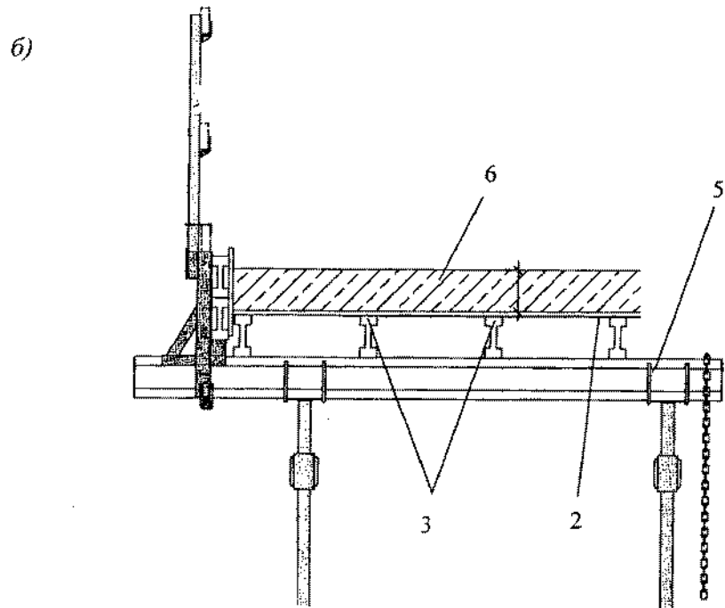
Рис. 22.17. Опалубка перекрытий фирмы «НОЕ» с балками Н20: а — общий вид; б — крайовой узел опалубки; 1 — балка Н20; 2 — опалубочный щит из водостойкой фанеры; 3 — продольная балка Н20; 4 — опорный штапик; 5 — вилка; 6 — бетонное перекрытие (до 30 см)
