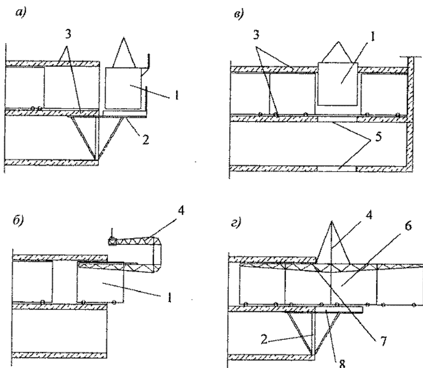
Рис. 23.4. Схема демонтажа объемно-переставной и туннельной опалубки:
