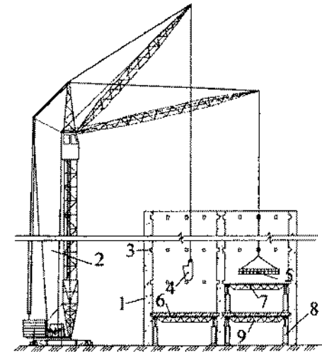
Рис. 24.5. Бетонирование междуэтажных перекрытий методом «снизу вверх»:
