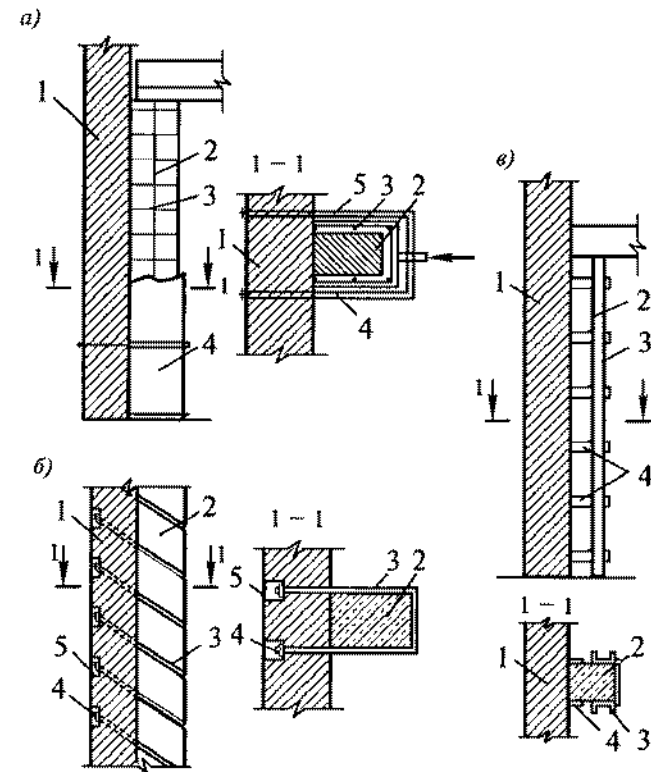
Р и с. 29.10. Усиление колонн, примыкающих к стенам:
