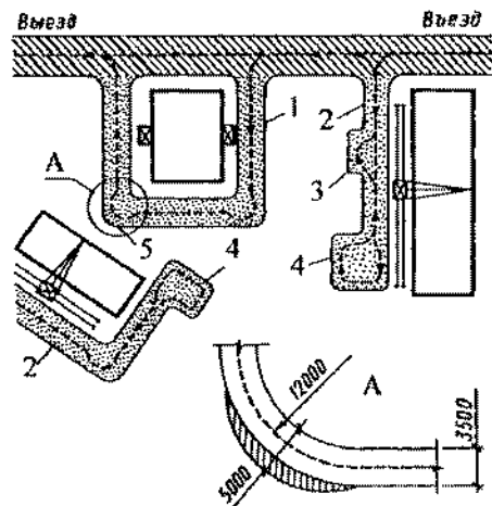
Рис. 3.2. Внутриплощадочные автомобильные дороги:
